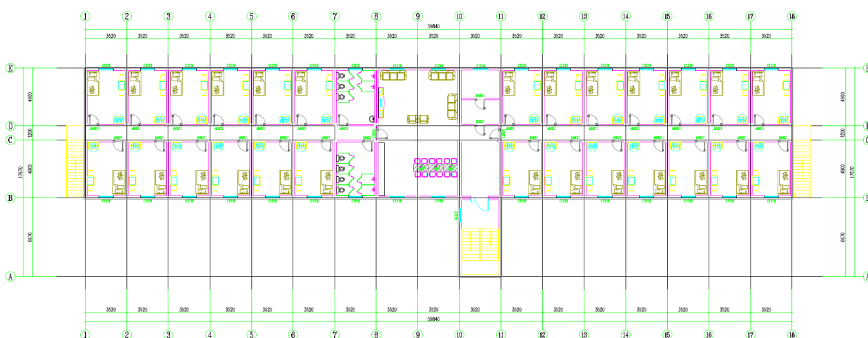
Pohjapiirroksat, 1 ja 2 kerros, 50 huonetta, 17,7 * 60 m
